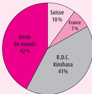
Répartition des envois en 2015 destinations principales
